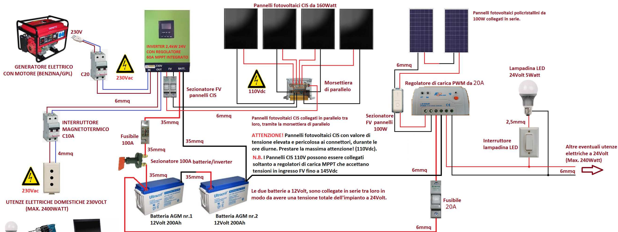
SCHEMA DI CABLAGGIO IMPIANTO FOTOVOLTAICO A ISOLA, CON BATTERIE A 24VOLT E INVERTER DA 2400WATT, REALIZZATO CON DUE TIPI DIVERSI DI PANNELLI (CIS E POLICRISTALLINI).
